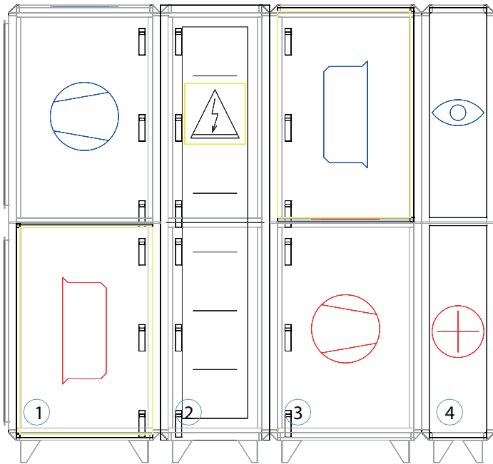
Maßstabelle für die Ausführung mit einem Rotationswärmetauscher (ER)
